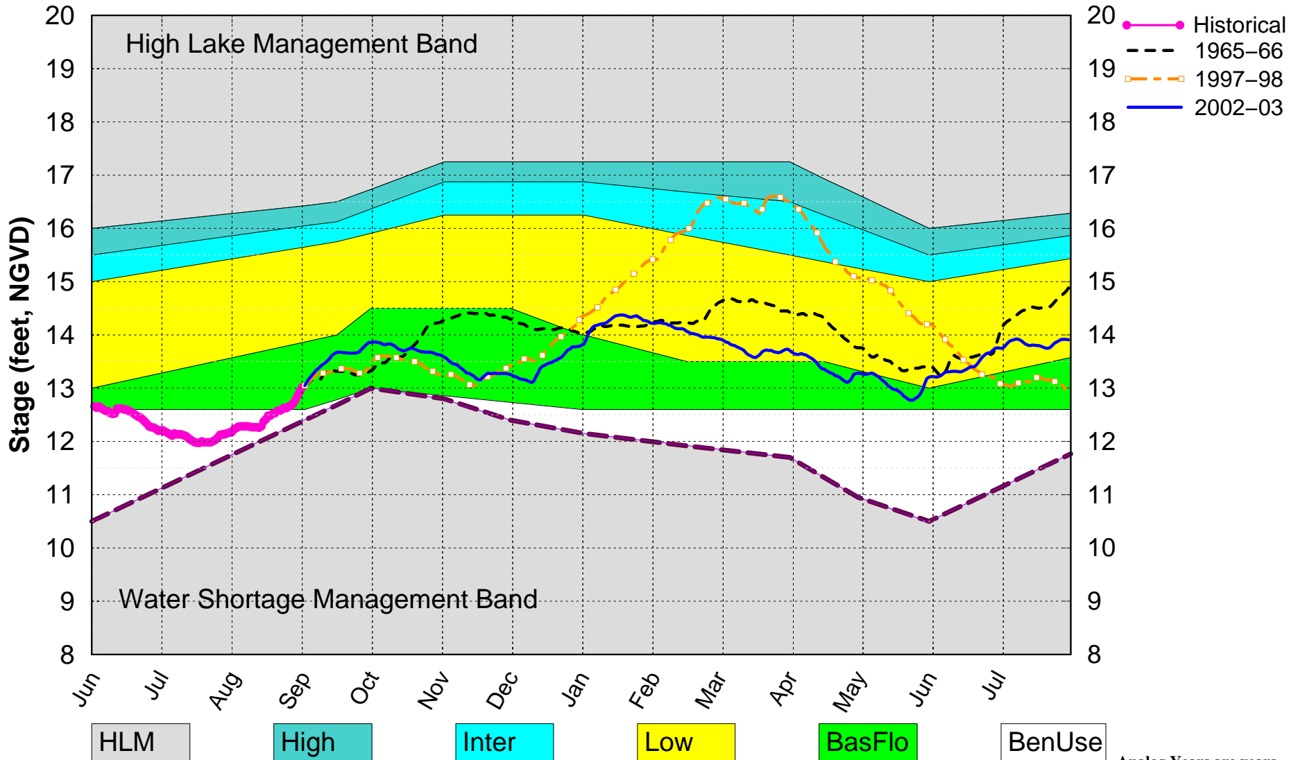
AMO Warm / El Nino Analog Years Plot PA_SEP15DPA
