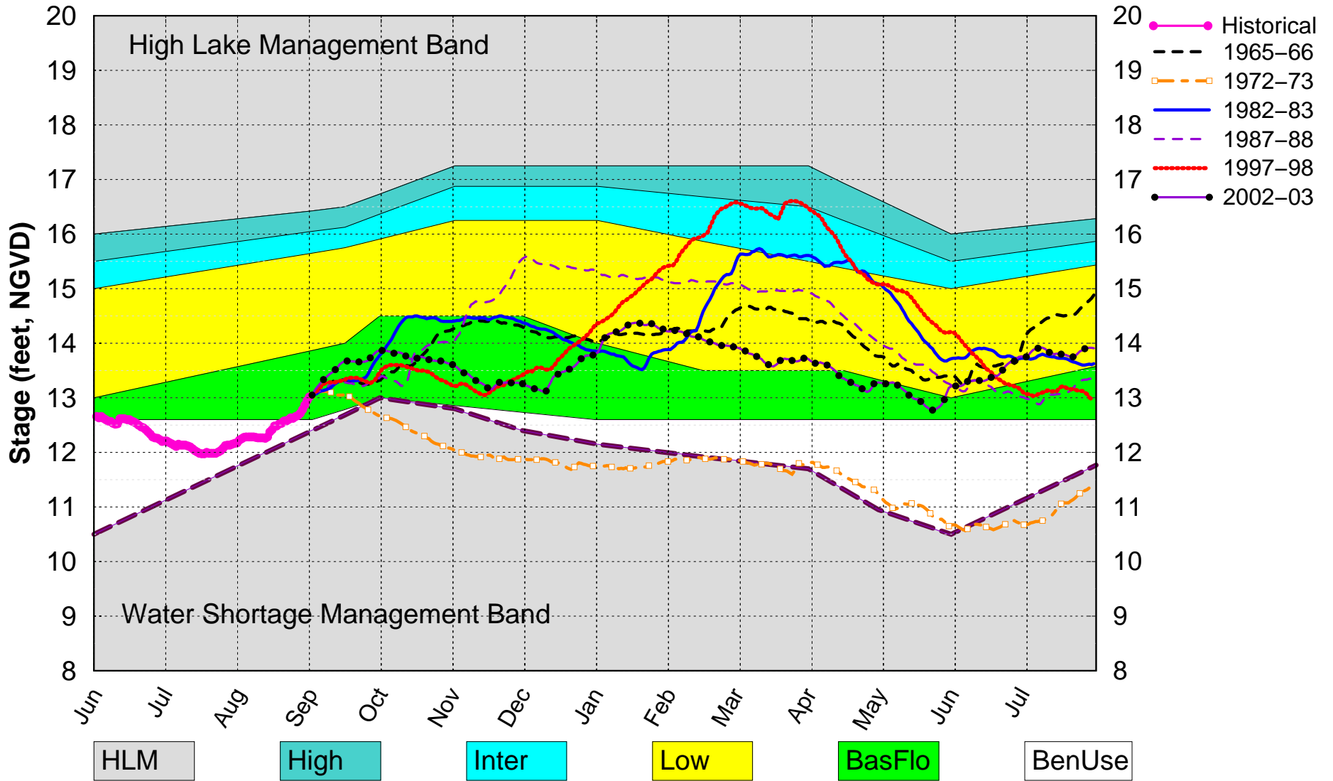
All El Nino Years Plot PA_SEP15DPA
